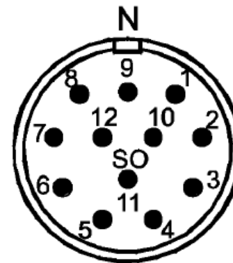
Face view of DIN M23 12C plug
